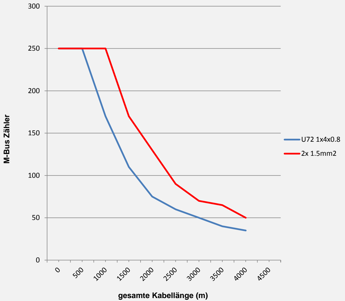
Anzahl der M-Bus Zähler in Abhängigkeit von der Leitungslänge
